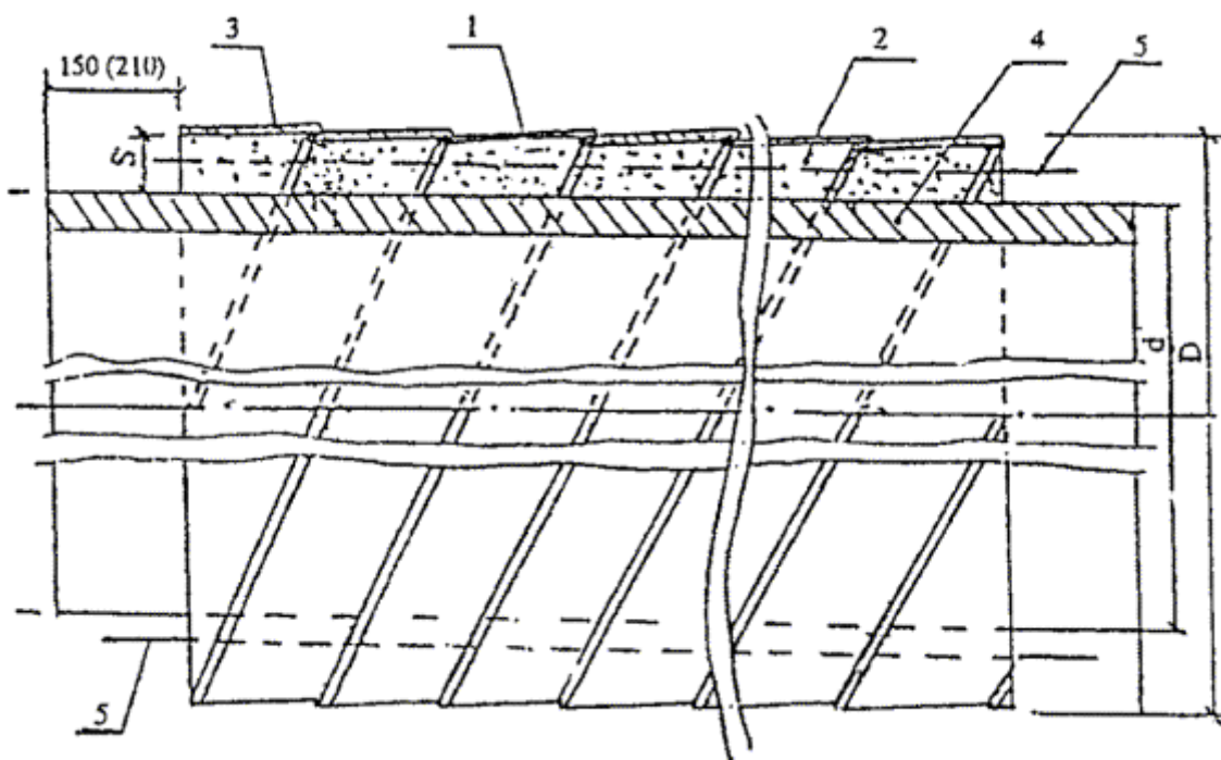
Рис. 2. Индустриальная конструкция труб с ППУ-ОЦМ изоляцией
