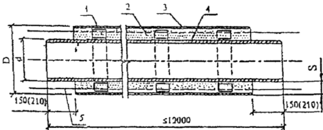
Рис. 1. Индустриальная конструкция труб с ППУ-ПЭ изоляцией
